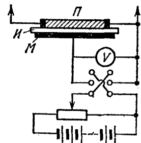
Рис. 10.9. Схема наблюдения стационарного эффекта поля.
