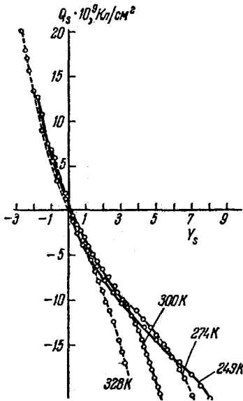
Рис. 10.10. Пример зависимости заряда поверхности от поверхностного потенциала для образца германия.
