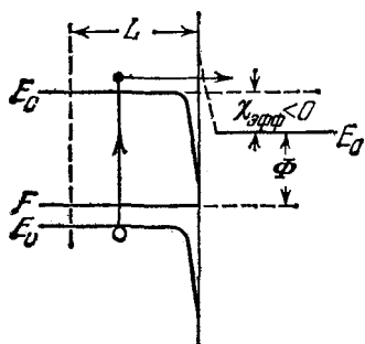
Рис. 10.17. Полупроводник с отрицательным эффективным электронным сродством.
