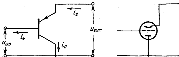
Рис. 8.9. Полупроводниковый триод в схеме с общим коллектором.
