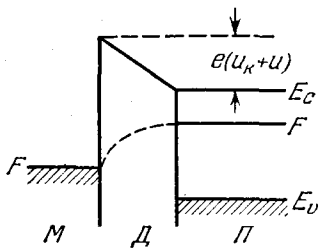
Рис. 6.16. Энергетическая диаграмма структуры металл — диэлектрик — полупроводник.
