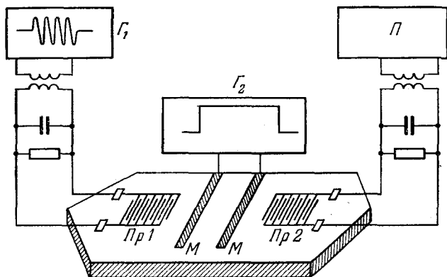
Рис. 15.10. Усиление поверхностных упругих волн дрейфом электронов. G_1 — импульсный генератор высокой частоты, G_2 — генератор прямоугольных импульсов ускоряющего напряжения, \Pi — радиоприемник, Пр1 и Пр2 — электромеханические преобразователи, М, М — металлические ускоряющие электроды.
