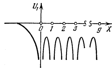
Рис. 10.2. Потенциальная энергия электрона в одномерной ограниченной решетке.
