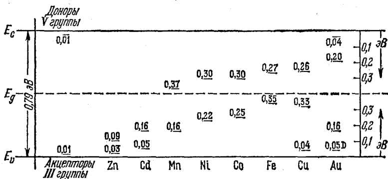
Рис. 2.20. Энергетические уровни некоторых примесей в германии при температуре абсолютного нуля. Все уровни — акцепторные, за исключением наинизшего уровня золота.
