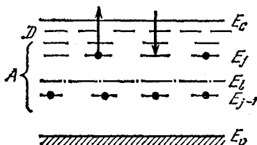
Рис. 5.13. Частично компенсированные многозарядные акцепторы. Полупроводник n -типа.
