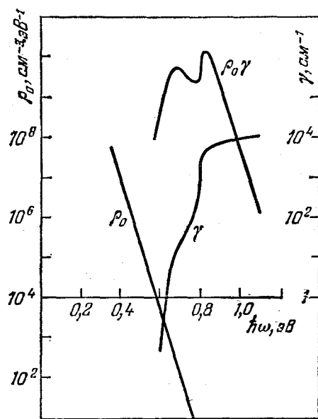
Рис. 9.3. К расчету коэффициента излучательной рекомбинации. Равновесная концентрация фотонов \rho_0 , коэффициент оптического поглощения \gamma и произведение \rho_0\gamma для германия при 300 К [2].
