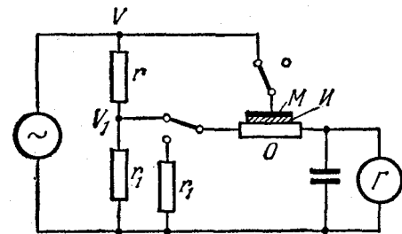
Рис. 10.13. Измерение частотной зависимости эффективной подвижности. O — образец, I — изолятор, M — металлическая обкладка, \Gamma — гальванометр.
