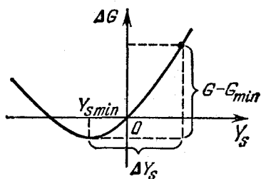
Рис. 10.8. К определению величины поверхностного потенциала.
