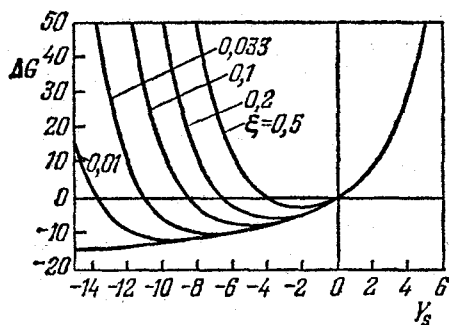
Рис. 10.7. Зависимость изменения проводимости \Delta G германия n -типа (произвольные единицы) от поверхностного потенциала Y_s = e\varphi_s/kT .
