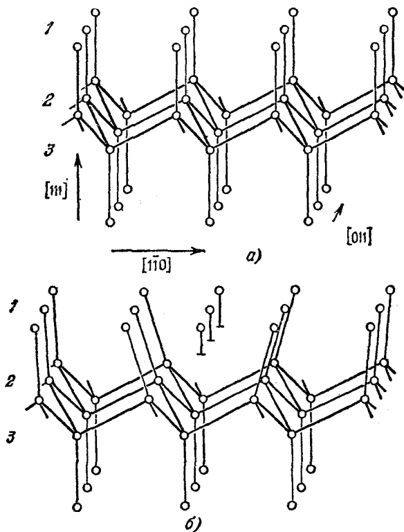
Рис. 2.25. а) Расположение атомов в структуре алмаза. б) Один из возможных типов линейной дислокации в структуре алмаза (по В. Шокли). Дислокация возникла вследствие частичного сдвига плоскости 1 относительно плоскости 2. Показаны также три атома на крае неполной атомной плоскости и их неспаренные, или «болтающиеся», связи.
