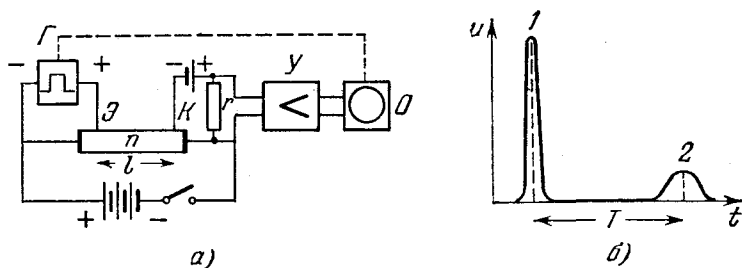
Рис. 7.13. Измерение скорости движения пакета инжектированных носителей.
