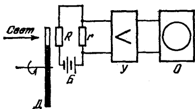
Рис. 7.4. Схема для наблюдения фотопроводимости.
