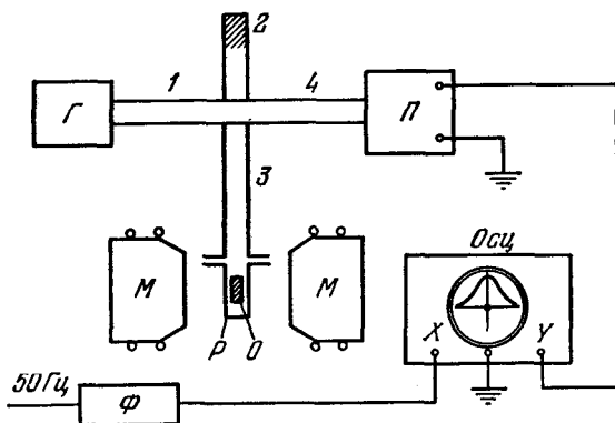
Рис. 4.4. Схема наблюдения диамагнитного резонанса. Г — генератор СВЧ колебаний, П — приемник, Осц — осциллограф, P — резонансная полость с образцом O, MM — электромагнит, Ф — фазовращатель.
