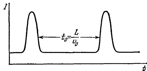
Рис. 16.15. Сила тока I в цепи нагрузки как функция времени t при движении доменов по образцу (схематически).
