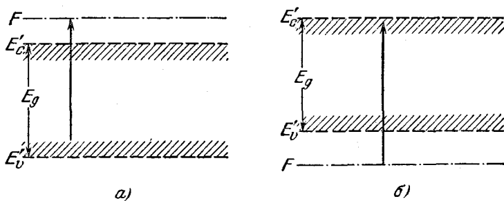
Рис. 19.8. Происхождение хвоста коэффициента поглощения в некомпенсированном полупроводнике. Заштрихованы области энергии, в которых плотность состояний на хвосте достаточно велика. Стрелкой указан один из возможных переходов, ответственных за поглощение фотонов с энергией, меньшей E_g . а) n -тип; б) p -тип.
