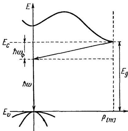
Рис. 18.6. Электронные переходы в многодолинном полупроводнике (германий) с участием фона.
