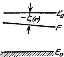
Рис. 6.2. К условию равновесия электронного газа.
