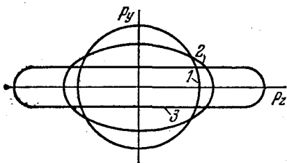
Рис. 16.4. Контуры постоянной функции распределения в пространстве квазиимпульсов. Ось Z направлена вдоль вектора напряженности электрического поля; оси Y и X (последняя не показана) эквивалентны. Кривая 1 изображает контур при \xi = 0 ; кривые 2 и 3 отвечают слабо и сильно неупругому рассеянию ( \eta \ll 1 и \eta \approx 1 ).
