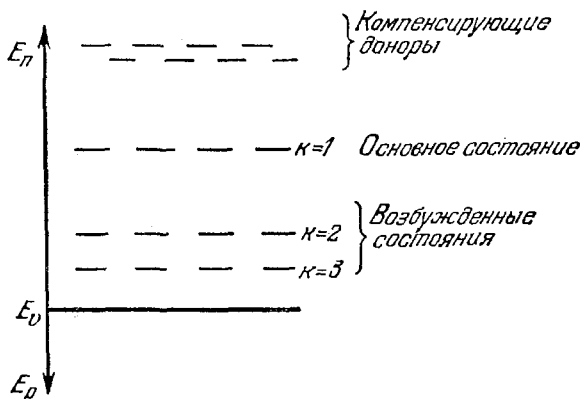
Рис. 5.6. Энергетический спектр связанной дырки при наличии возбужденных состояний.
