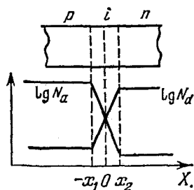
Рис. 7.8. p — n -переход.
