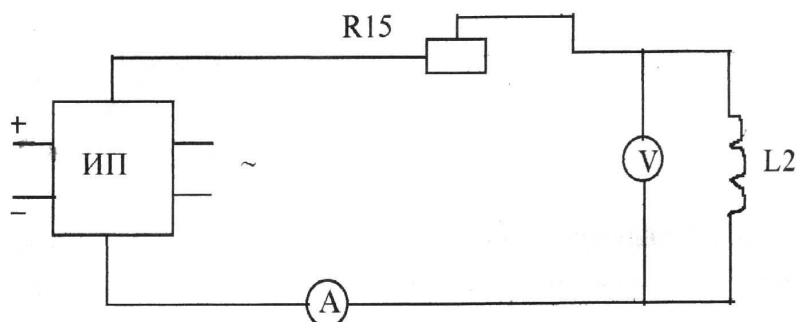
Рис. 1. Принципиальная схема для определения L .
