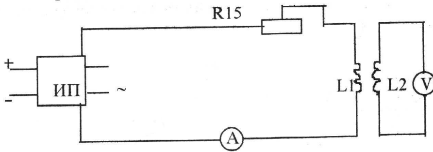
Рис 2 Принципиальная схема для определения взаимной индуктивности
